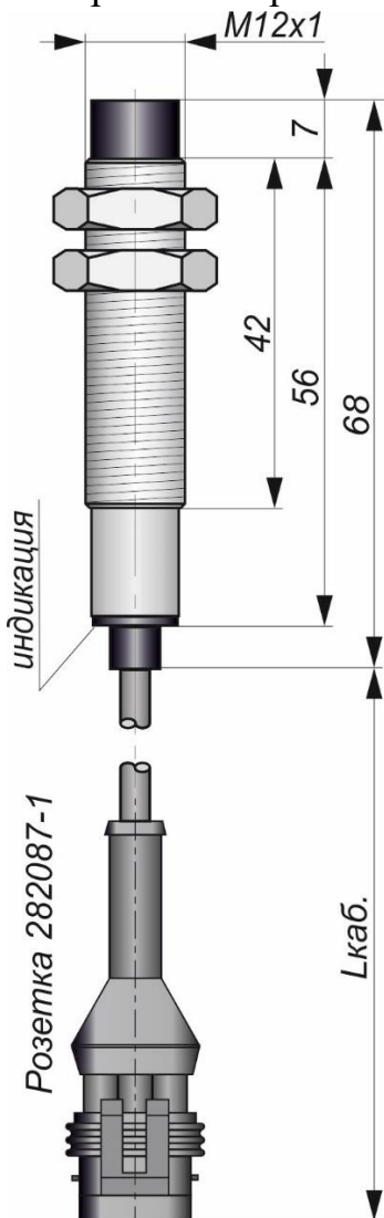
Габаритный чертеж
