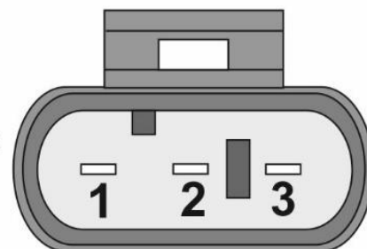
Нормально-разомкнутый контакт
